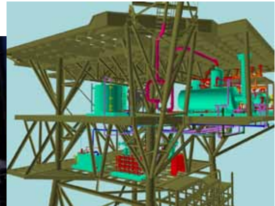
BPZ Plataforma Albacora - Ingeniería y gestión del proyecto Offshore Tumbes, Perú 10.000 BPD EPCm / 2011
